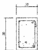
Detalhe da viga Baldrame ESCALA: 1:10
