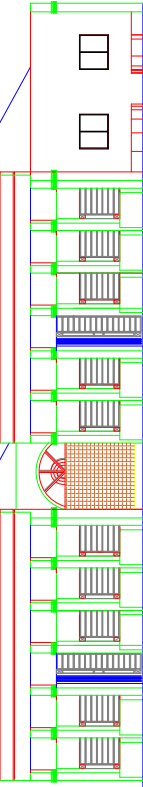
07 FACHADA FINAL ESCALA 1/100
