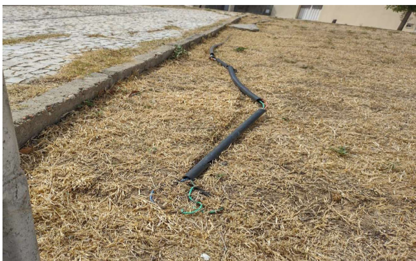
FOTO 10 – INSTALAÇÕES ELÉTRICAS DANIFICADAS (ELETRODUTOS EXPOSTOS, QUEBRADOS EM VÁRIOS LOCAIS E FIAÇÕES EXPOSTAS, DESEMCAPADAS E QUEBRADAS DEVIDO A EXPOSIÇÃO AO SOL).
