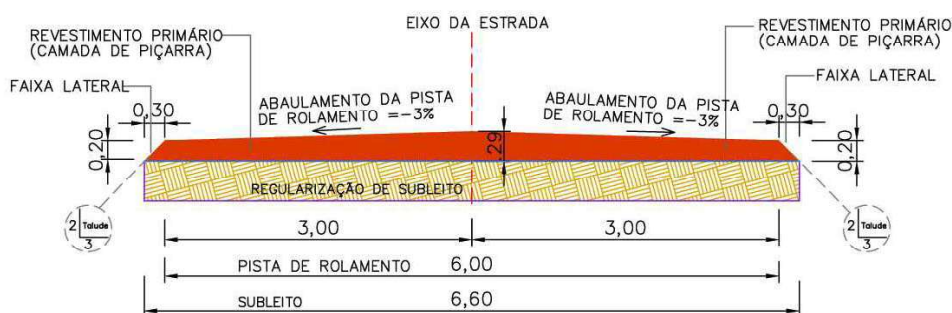
SEÇÃO TRANSVERSAL EM ATERRO ESC. 1/50
