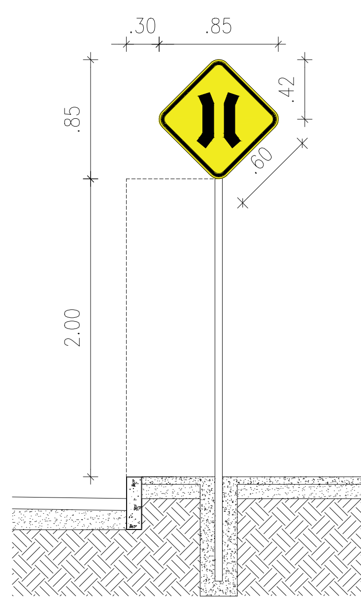
04 DETALHE DA PLACA SEM ESCALA
