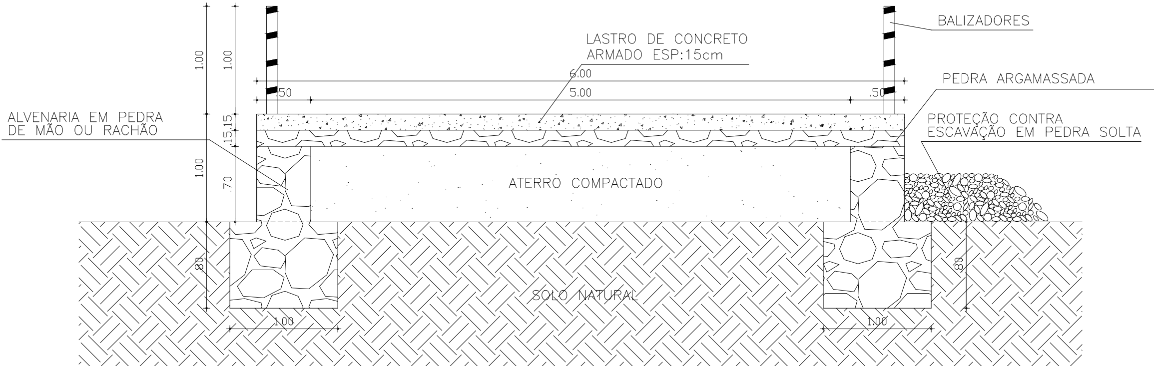
04 CORTE TRANSVERSAL DD
