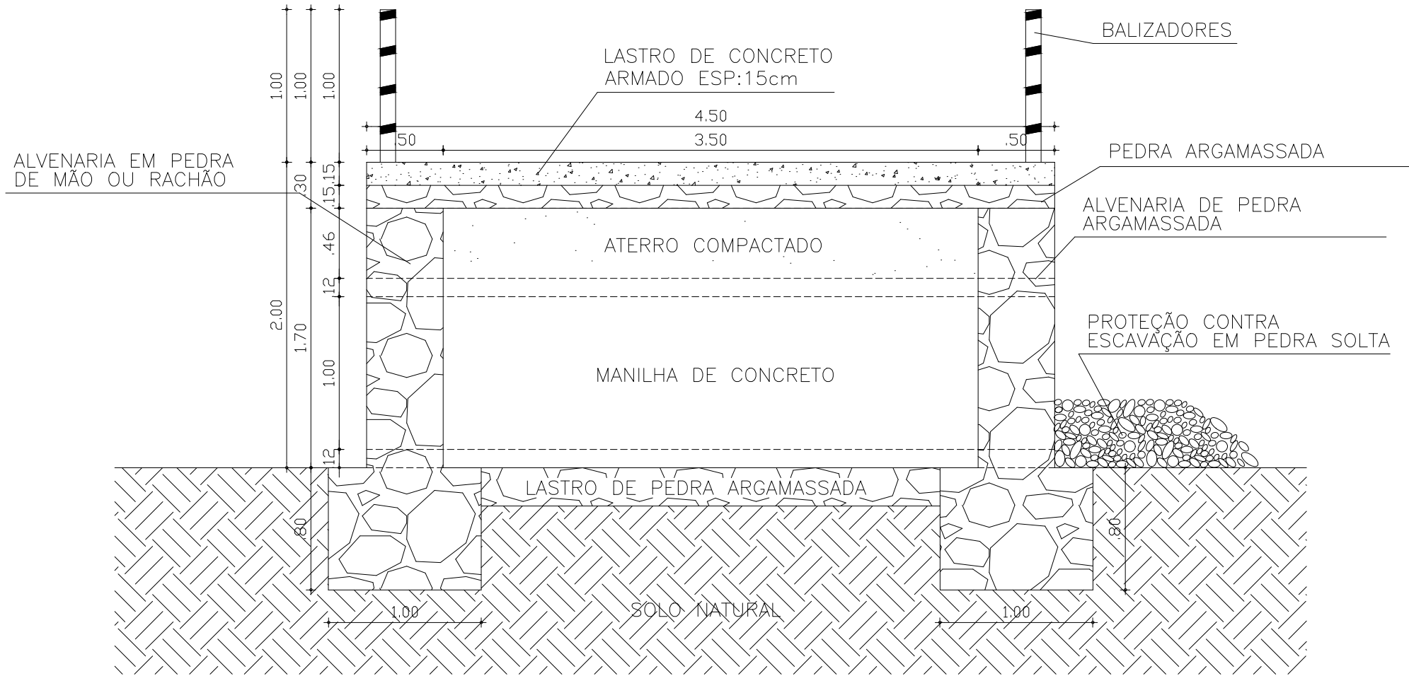
02 CORTE TRANSVERSAL BB
