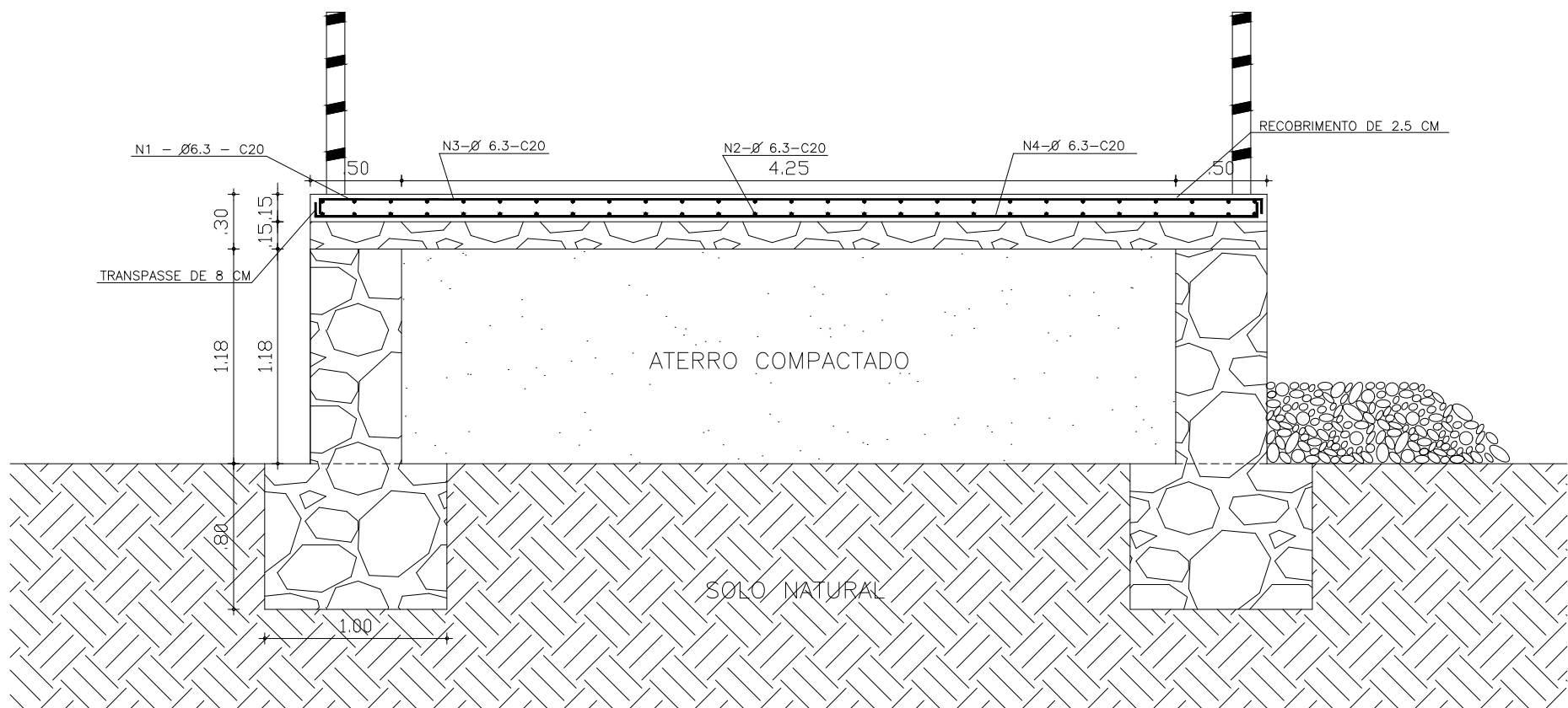
05 DETALHE DA ARMADURA
