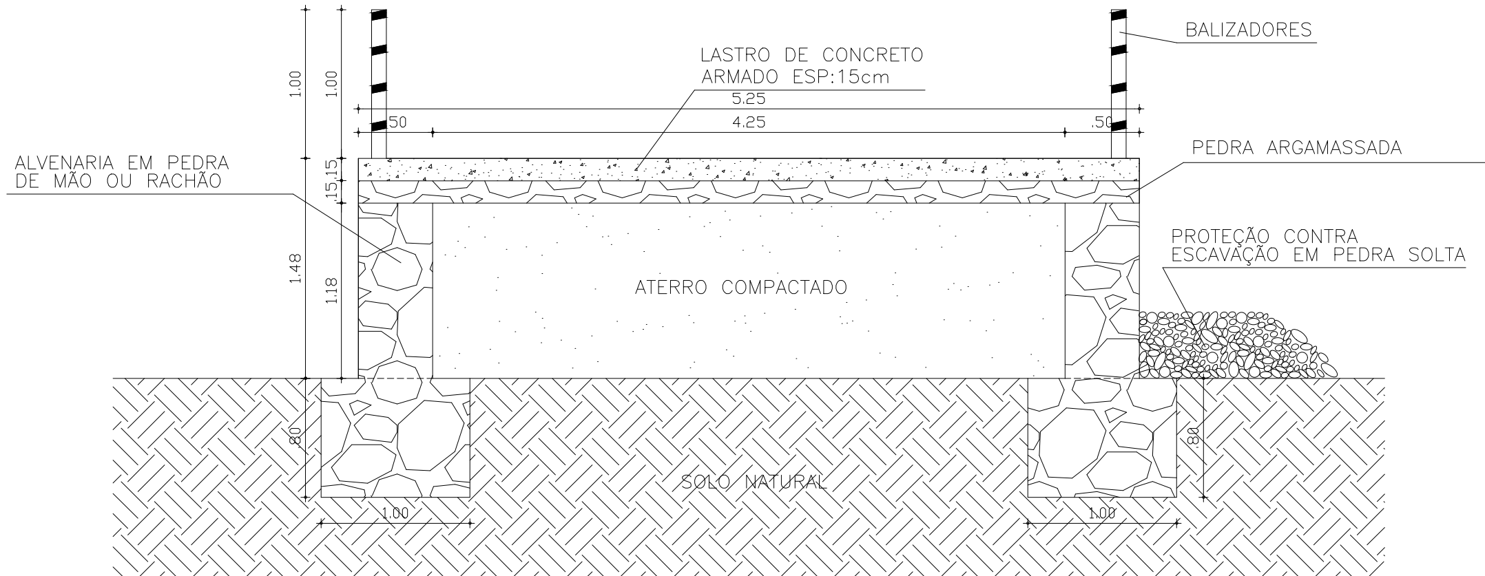
03 CORTE TRANSVERSAL CC
