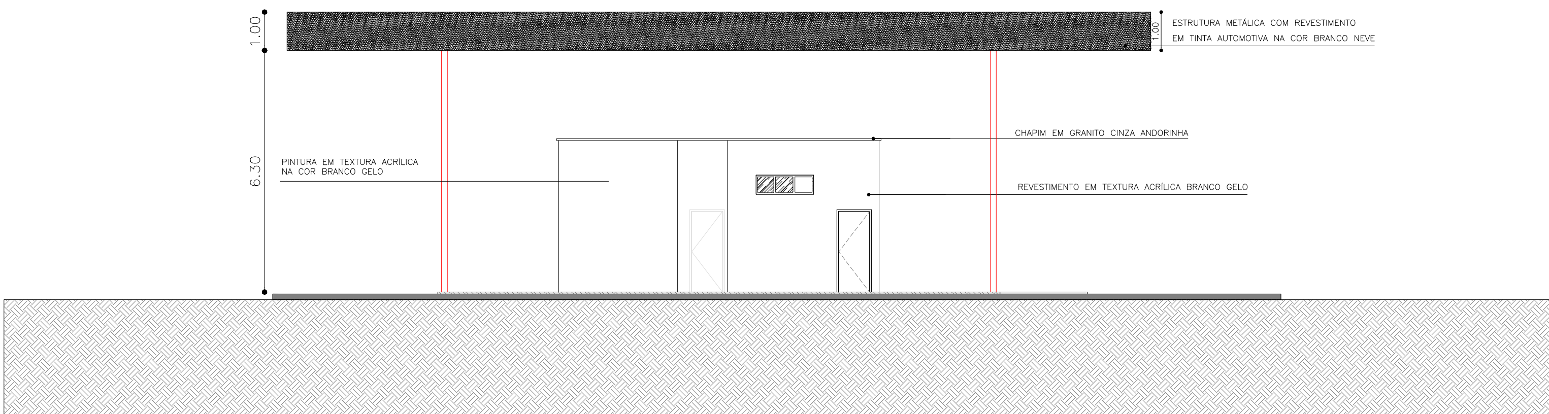
04 FACHADA 04 ESC. 1/100
