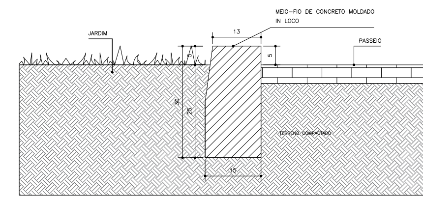
04 DETALHE - MEIO FIO INTERNO
