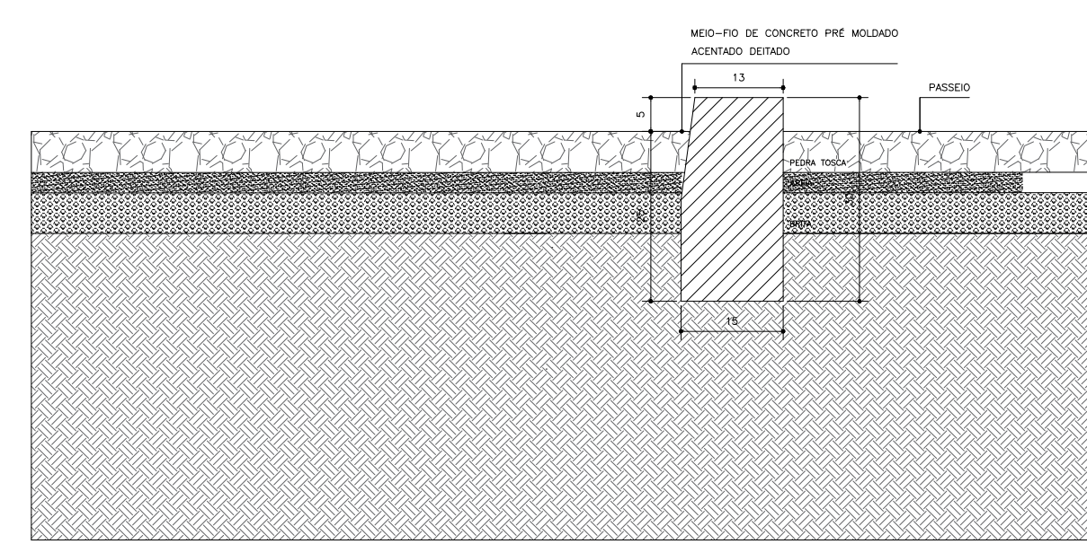
03 DETALHE - MEIO FIO EXTERNO
