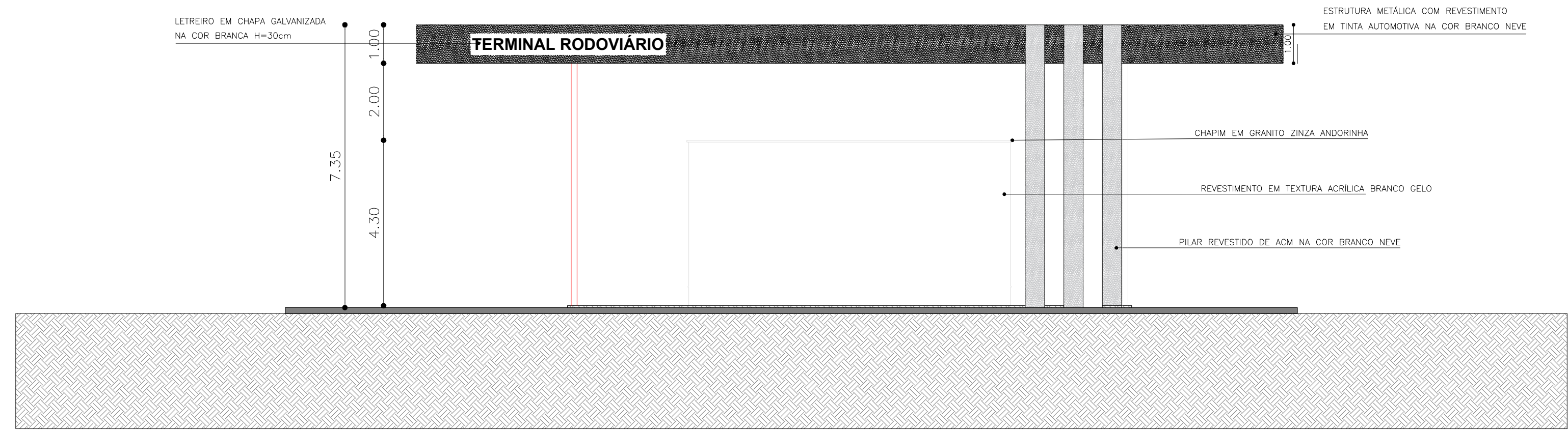
01 FACHADA PRINCIPAL 01 ESC. 1/100
