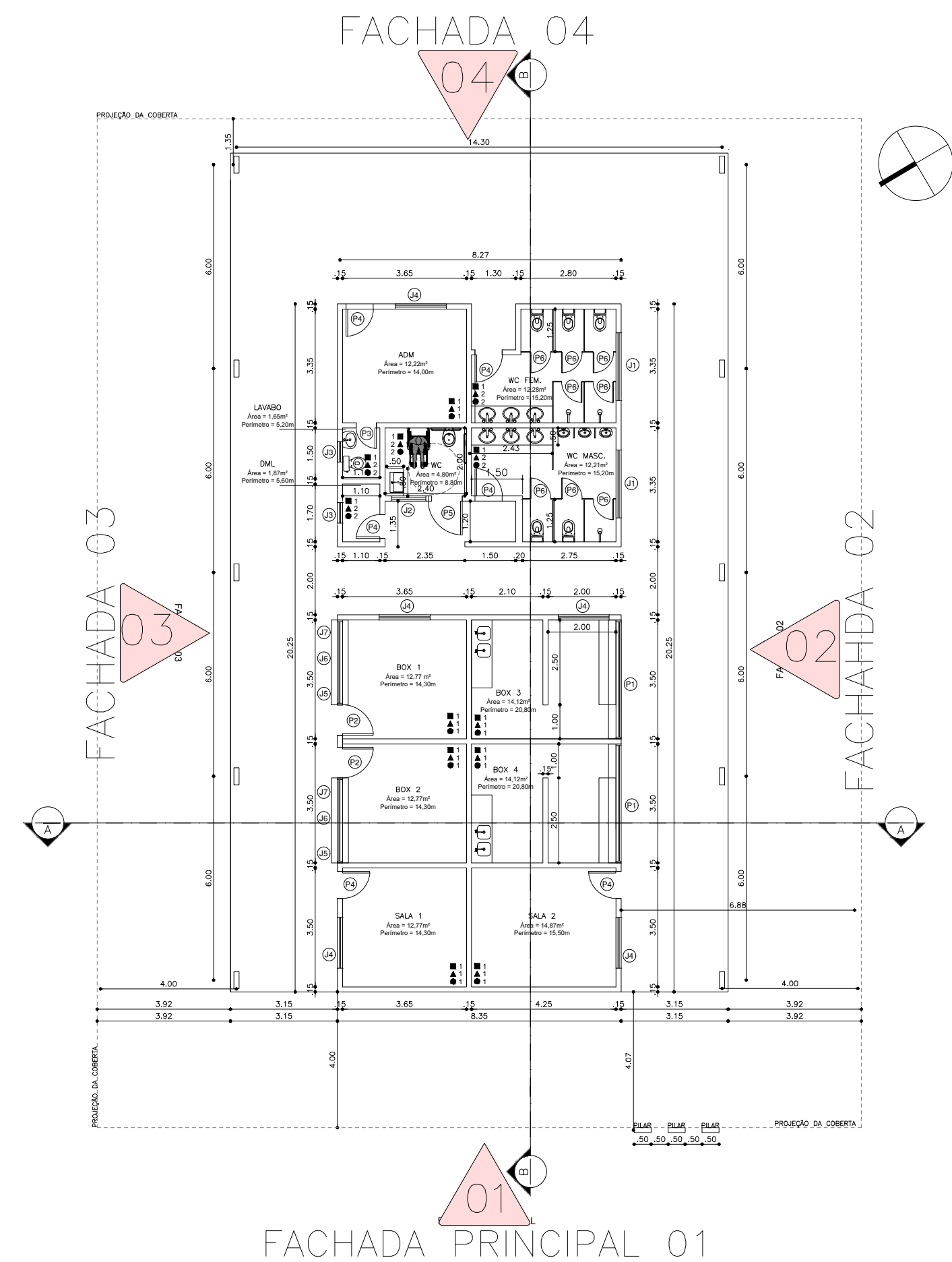
05 PLANTA BAIXA ESC. 1/75
