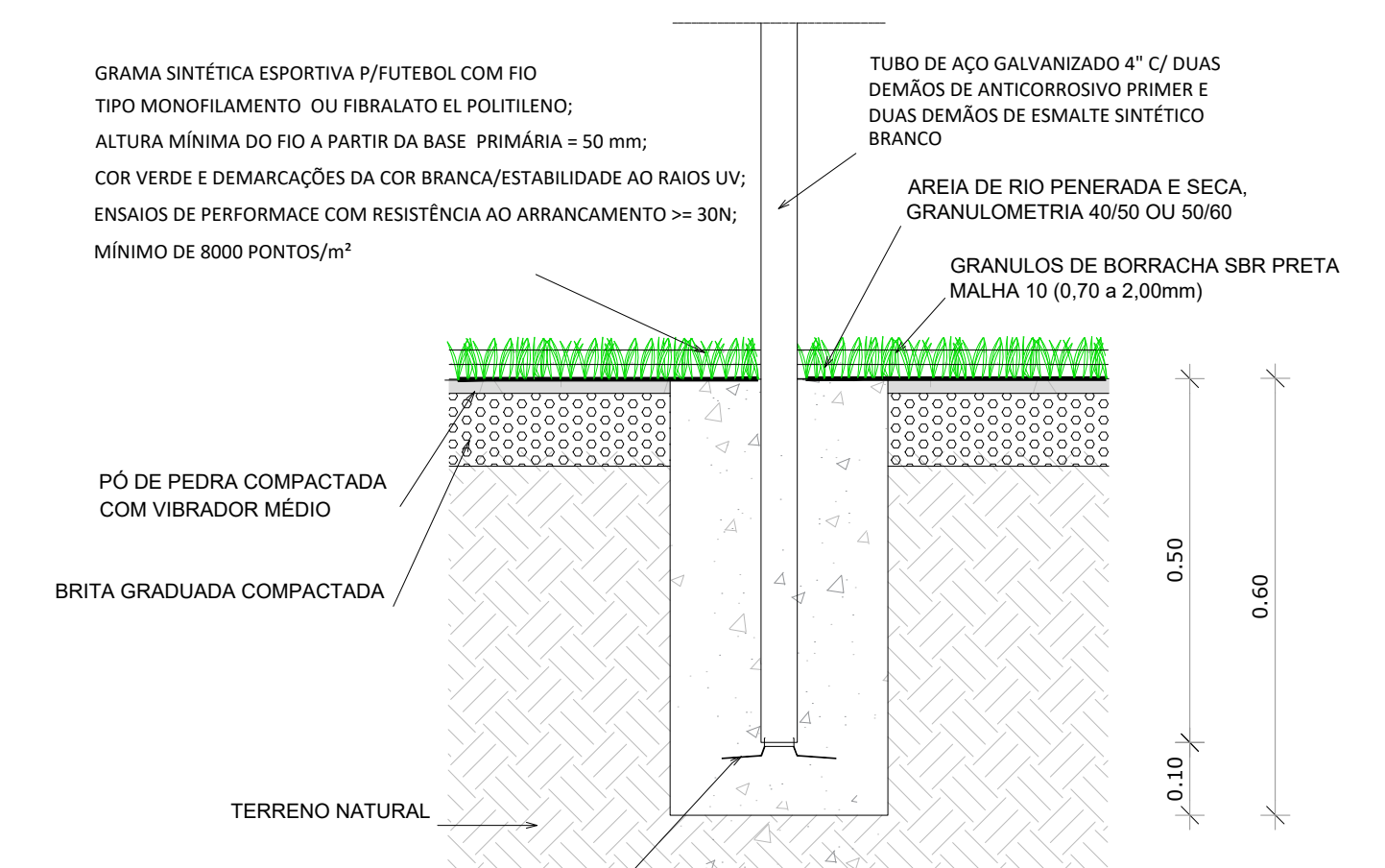
06 DET. - CHUMBAMENTO DA TRAVE Esc. - 1:25
