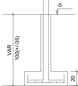
CORTE ESC 1:25
