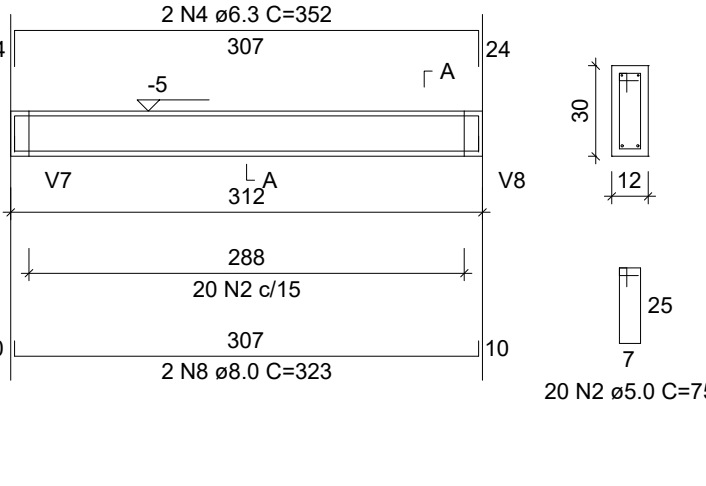
V2 ESC 1:50
