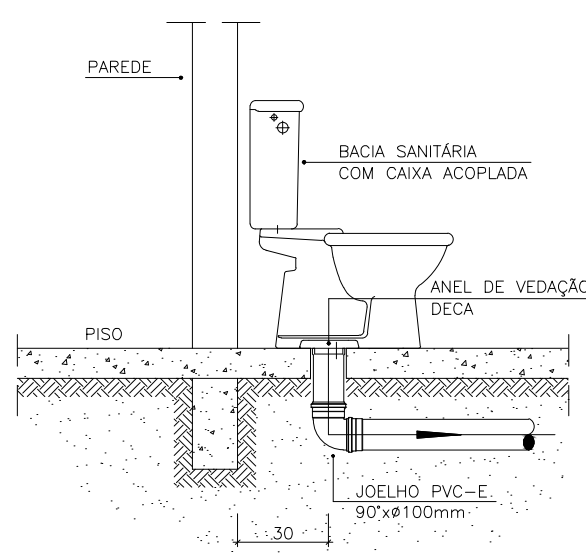
DETALHE GENÉRICO DO VASO SANITÁRIO
