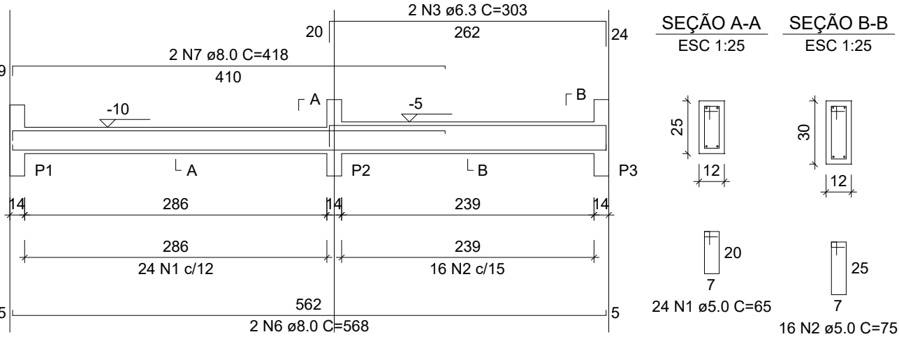
V1 ESC 1:50
