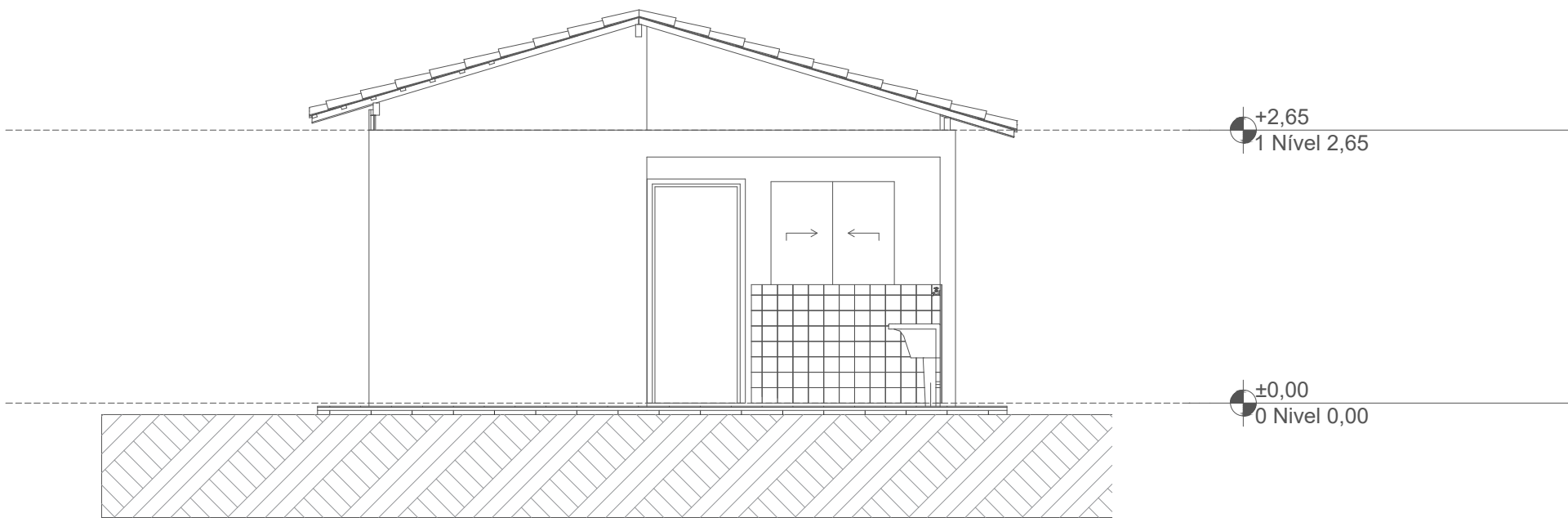
03 VISTA 3 ESC.: 1/60
