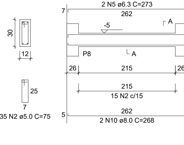
V4 ESC 1:50
