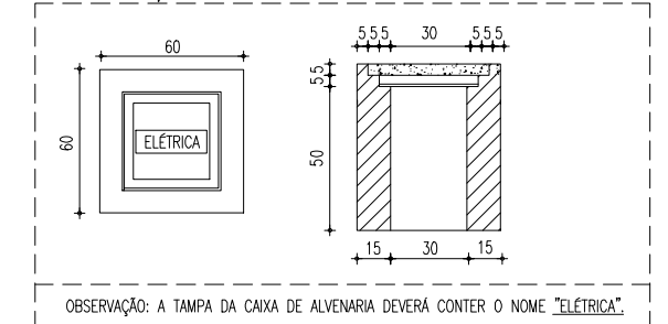
DETALHE-CAIXA DE ALVENARIA 30x30x50cm escala: s/e
