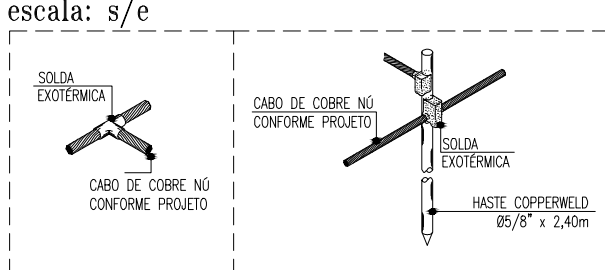
DETALHE-SOLDAS EXOTÉRMICAS escala: s/e
