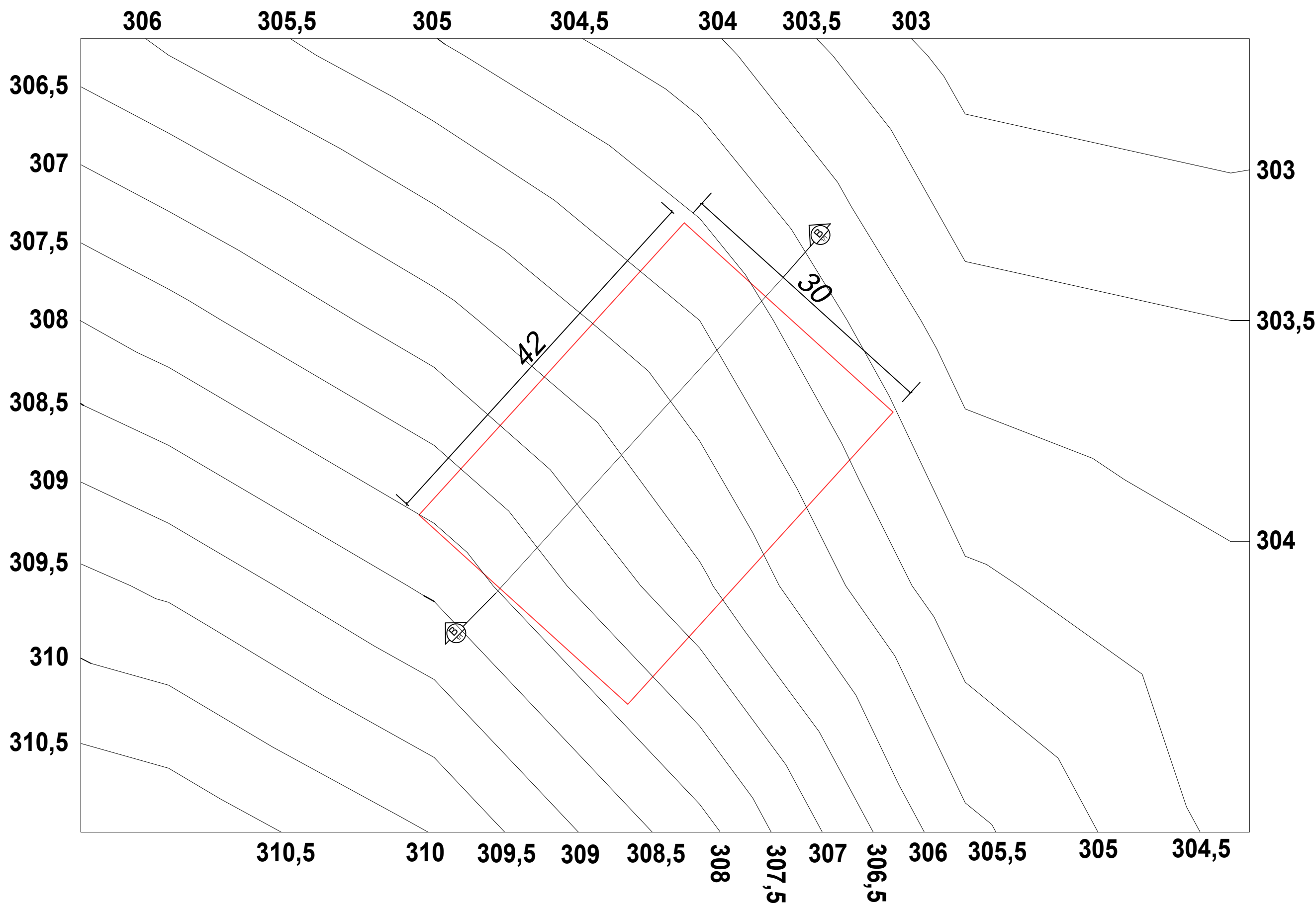
04 PLANTA DE TOPOGRAFIA ESC.: 1/400
