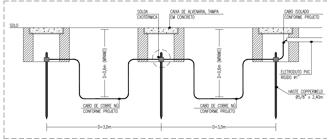
DETALHE-MALHA DE ATERRAMENTO escala: s/e
