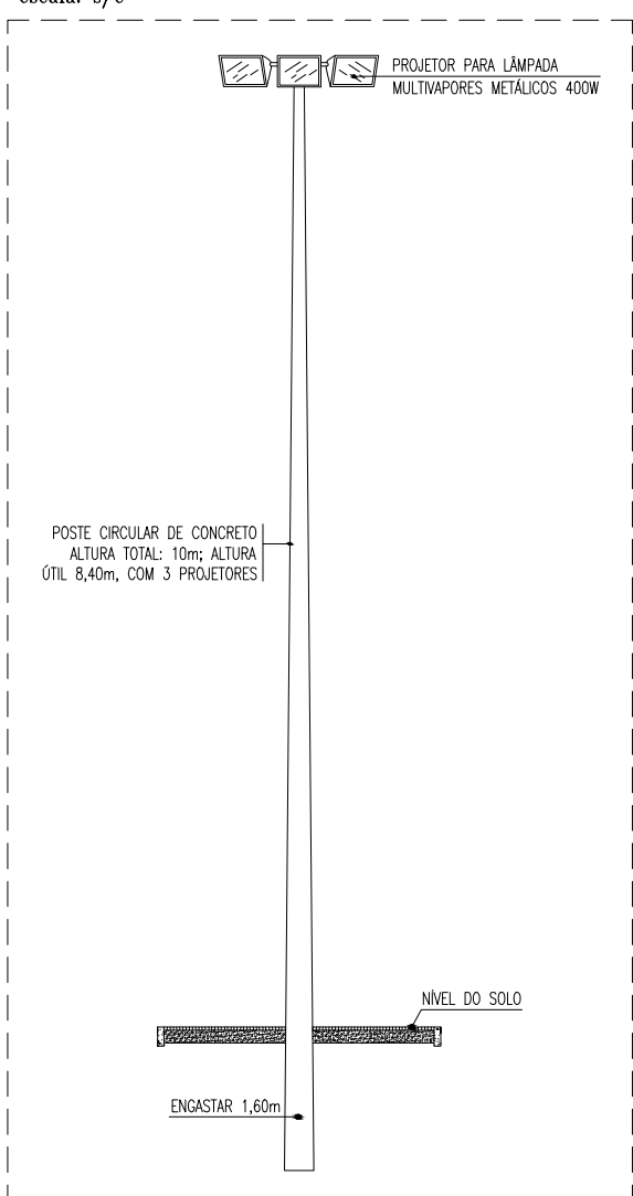
DETALHE - POSTES 10m escala: s/e
