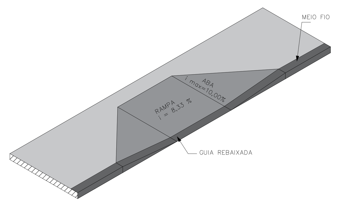
04 DET. - 03 RAMPA PESPECTIVA Esc. - 1:35
