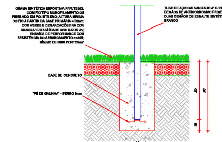
04 DET. CHUMBAMENTO TRAVE
