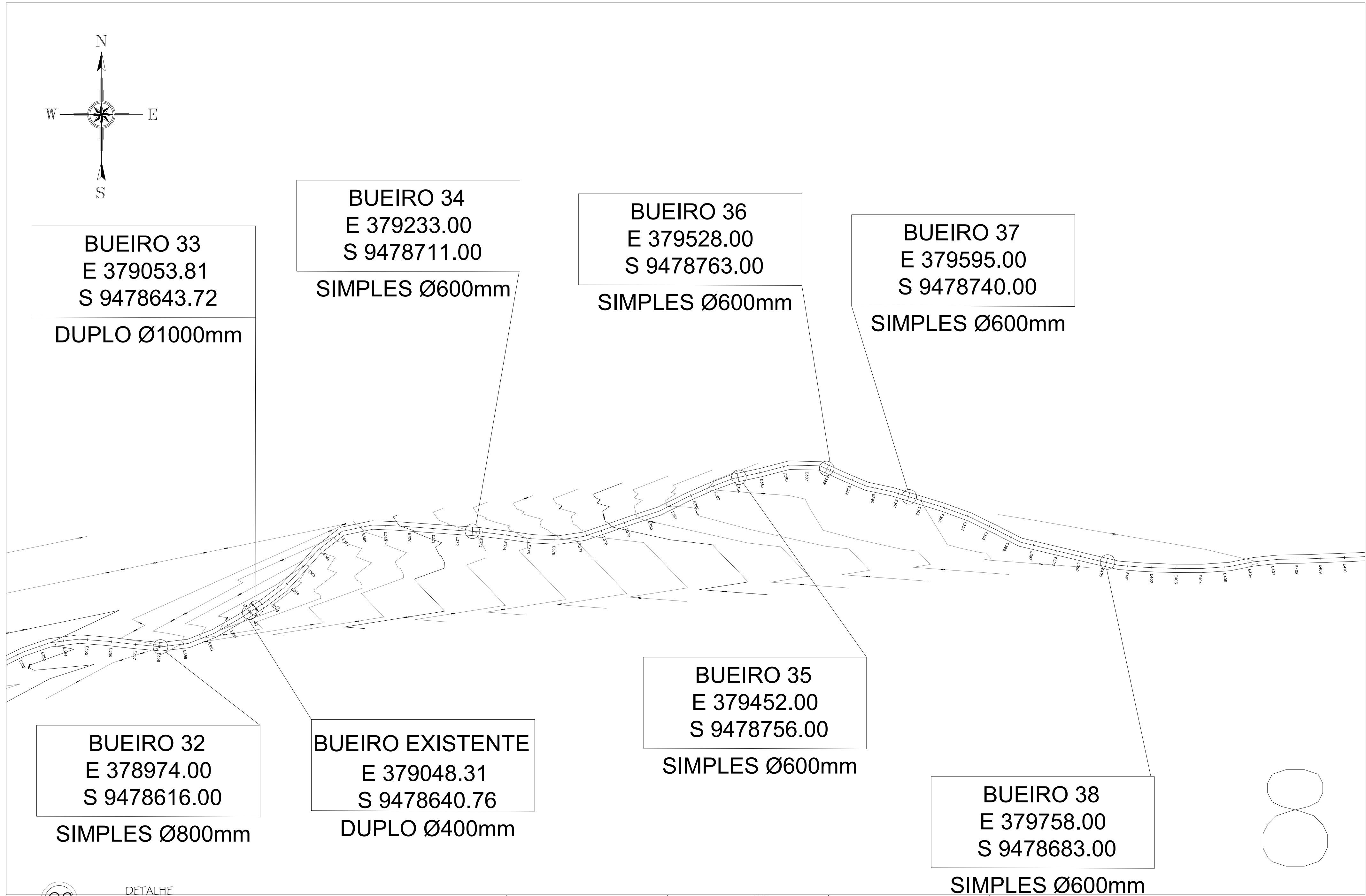
02 DETALHE ESC.: 1/2000
