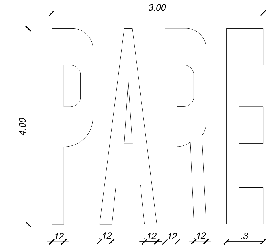
02 DET. LEGENDA NO SOLO 'PARE' SEM ESCALA
