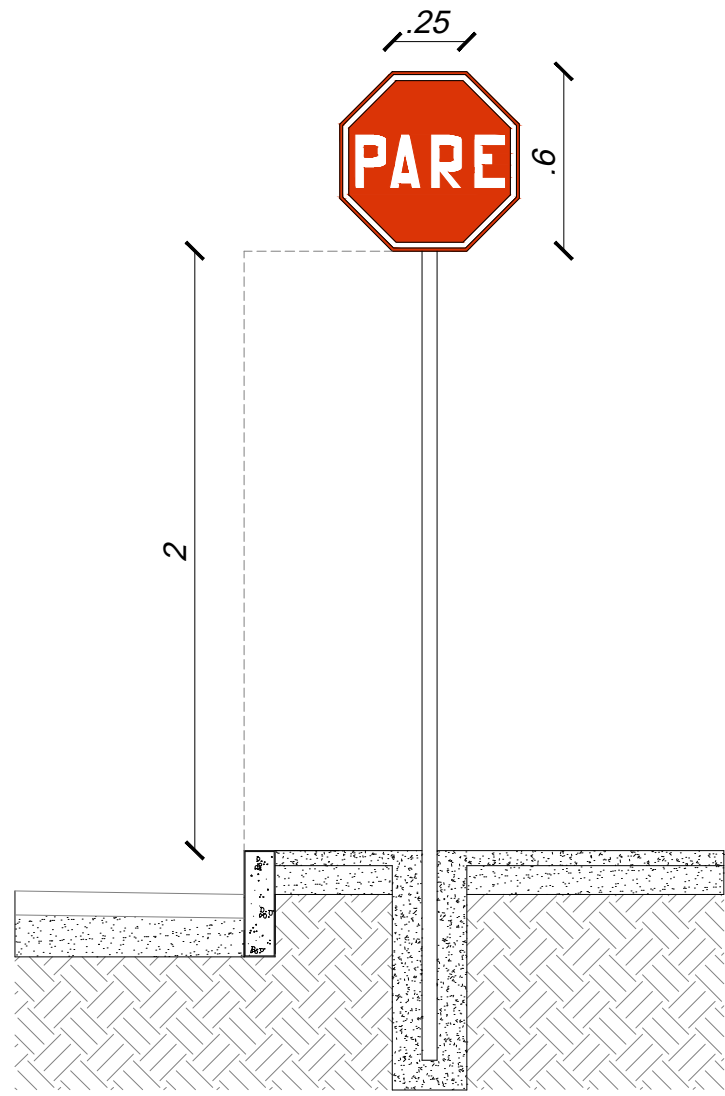
01 DETALHE DAS PLACAS SEM ESCALA
