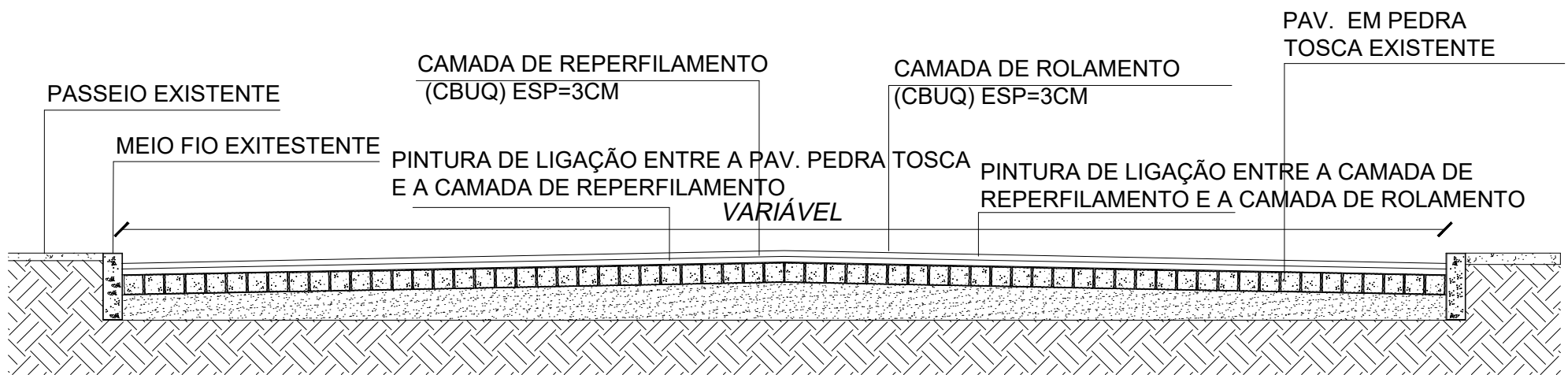
04 DETALHES DO CAP. ASFÁLTICO SEM ESCALA
