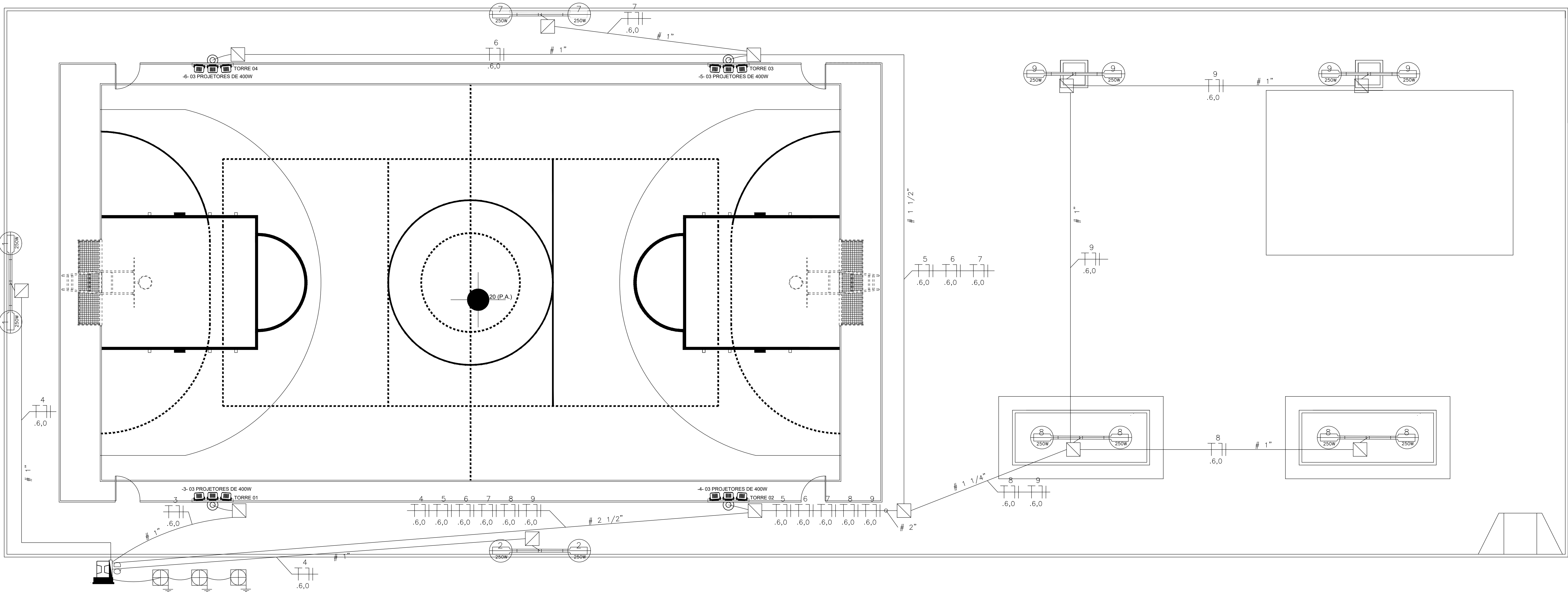
01 PROJETO ELÉTRICO ESC.: 1/75
