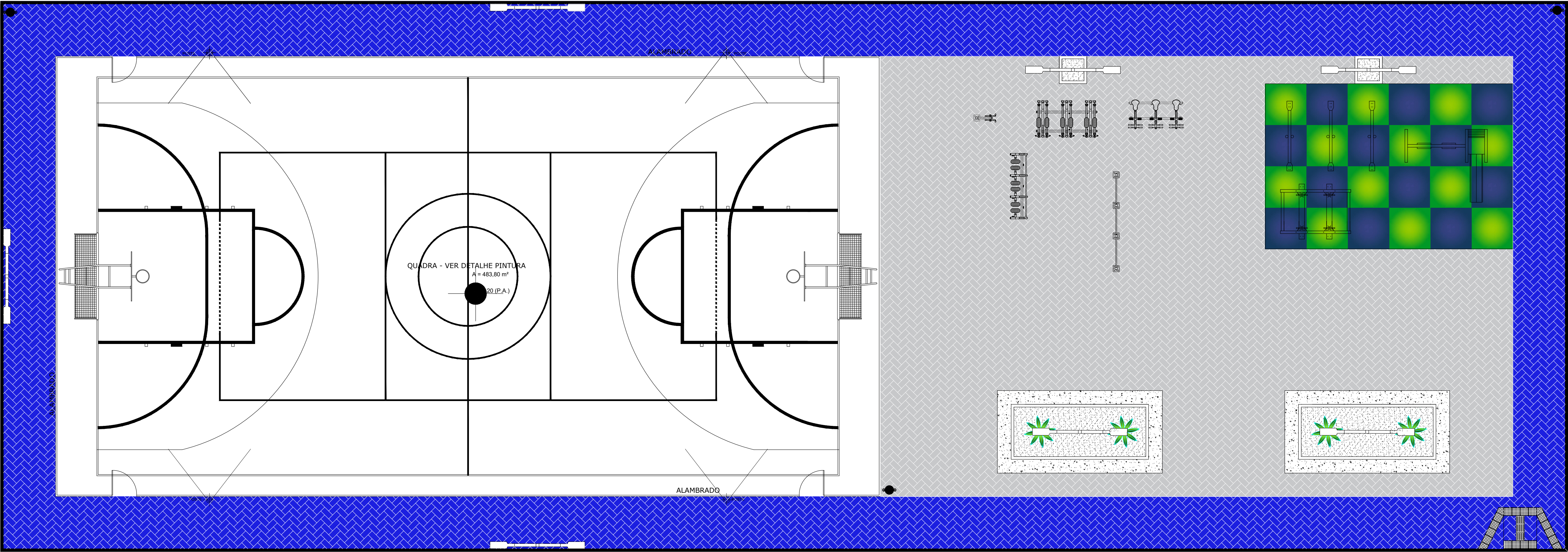
01 PLANTA DE LAYOUT ESCALA: 1/100
