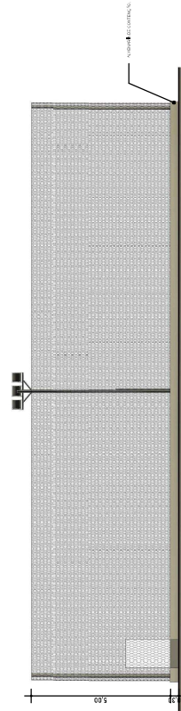
2 CORTE ARENINHA Escala - 1 : 100
