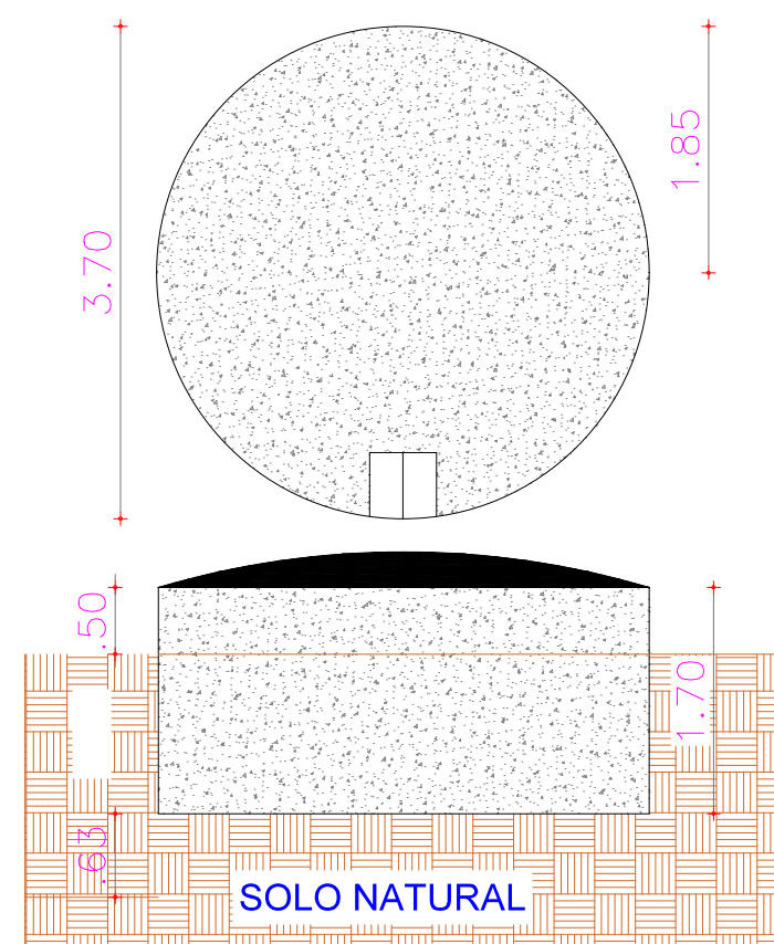
5 ESCOLA MARIA DIOGENES SALDANHA ESCALA 1/100
