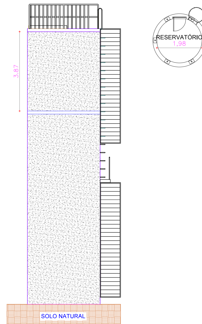
8 ESCOLA MARIA MONICA MAIA BARBOSA ESCALA 1/100
